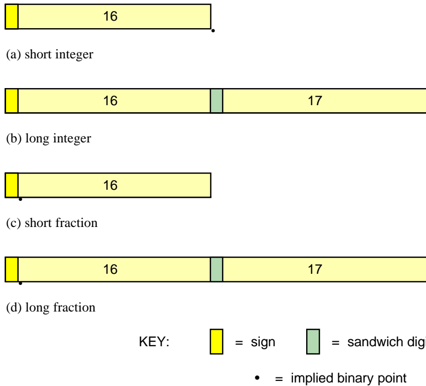
Fig. 6 Number formats
